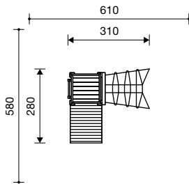
2.12120 huttencombinatie 212
