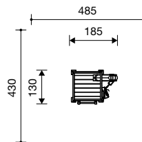
2.13400 huttencombinatie 340
