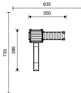
2.12170 huttencombinatie 217
