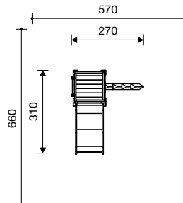
2.12170 huttencombinatie 217
