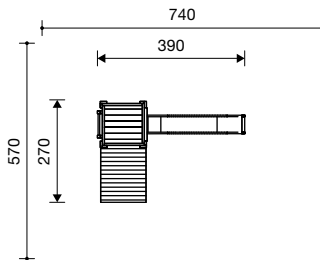
2.12160 huttencombinatie 216
