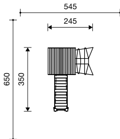
2.12160 huttencombinatie 216
