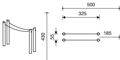
3.68500 dubbele hangkabel
