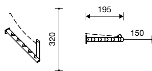
3.69520 klimstam met dubbele kettingleuning
