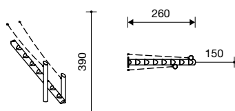
3.69520 klimstam met dubbele kettingleuning
