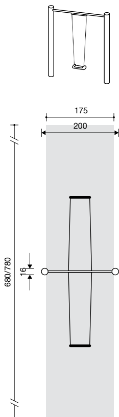
5.52125 hoge kleuterschommel
