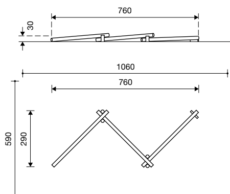
6.72110/6.72115 driedelige evenwichtsbalk
