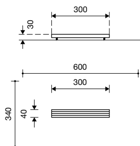
6.73110/6.73115 verende evenwichtsbalk
